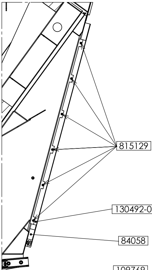
SECTION G-G SCALE 1 : 15
