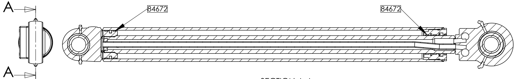
SECTION A-A SCALE 1 : 5
